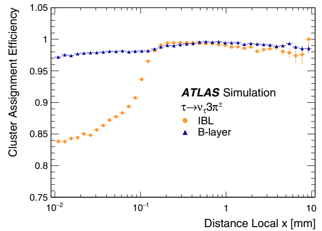
(d) \tau \rightarrow \pi^+\pi^-\pi^+\nu_\tau sample
